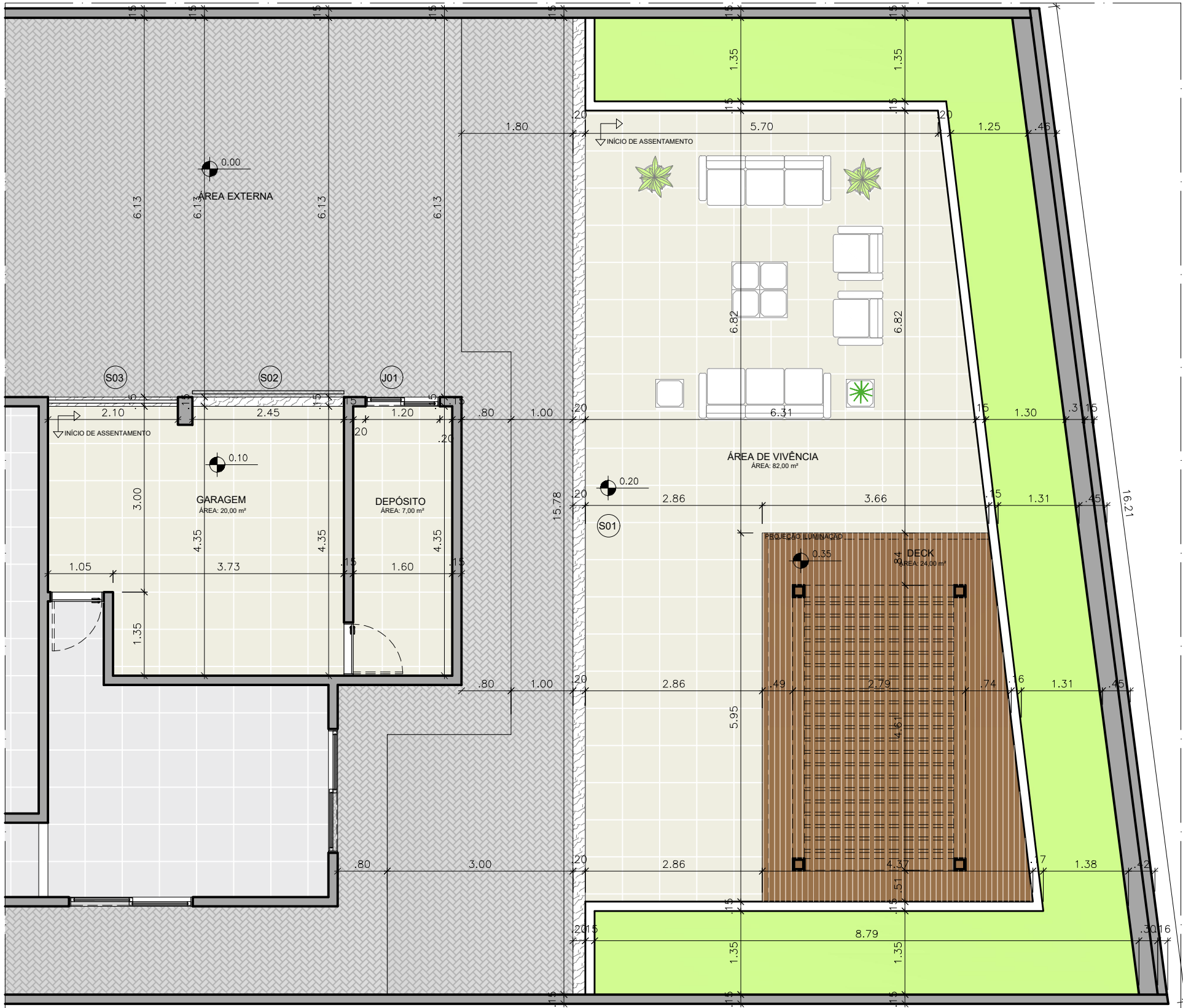
PRETENDIDA (PLANTA BAIXA - TÉRREO)
